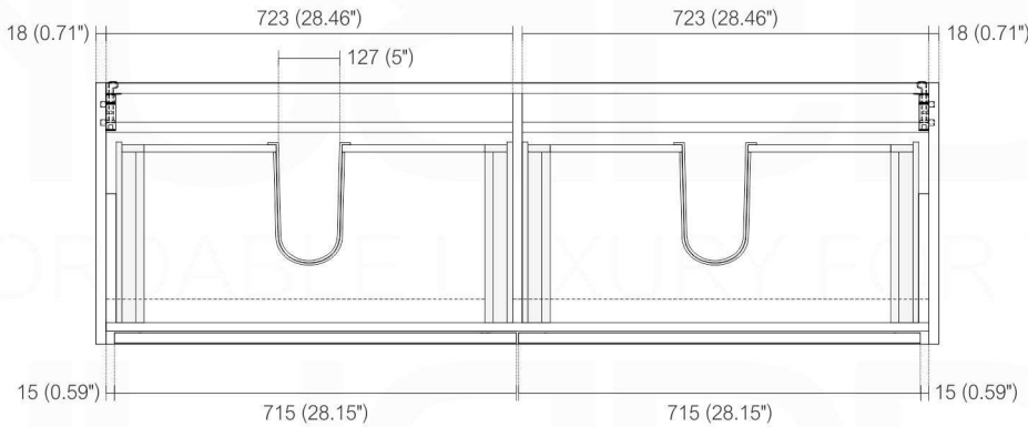
. TOP ELEVATION
