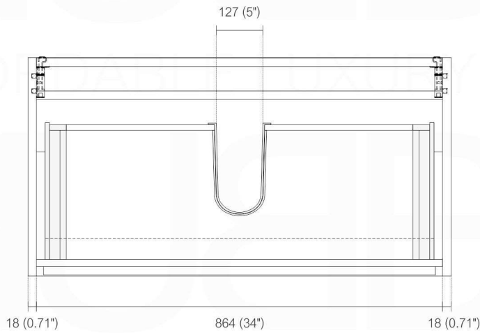
TOP ELEVATION
