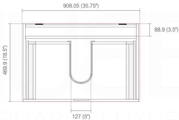
. TOP ELEVATION
