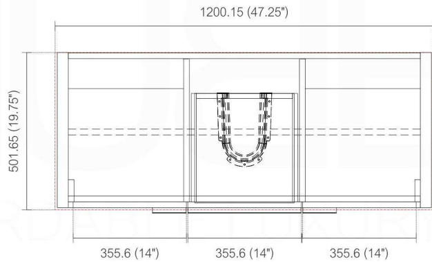
TOP ELEVATION
