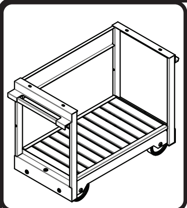
Fig 3 : Coloque el cuerpo de la parrilla sobre la base previamente armada y fije los bulones , con sus arandelas correspondientes, a las tuercas remachadas ubicadas en la base .
