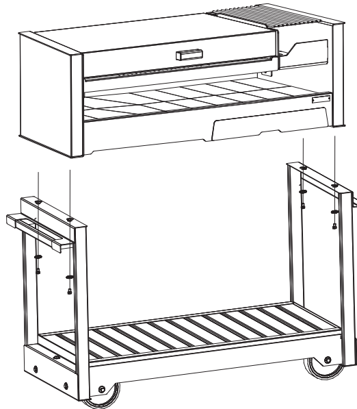
Fig 3 : Coloque el cuerpo de la parrilla sobre la base previamente armada y fije los bulones , con sus arandelas correspondientes, a las tuercas remachadas ubicadas en la base .
