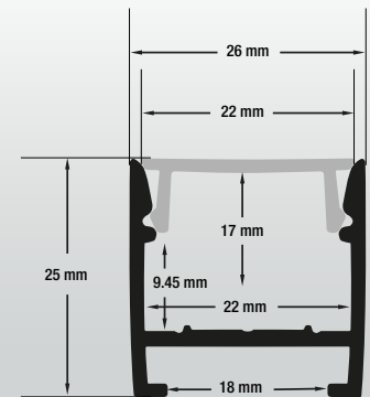
Model: VBD-CH-RH4
