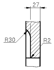
B-B 剖面
