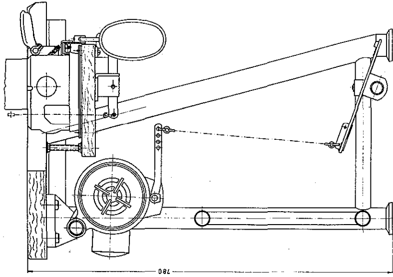
Schnitt A-B
