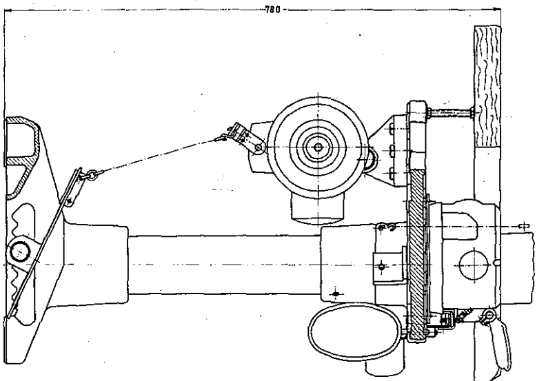
Schnitt A-B
