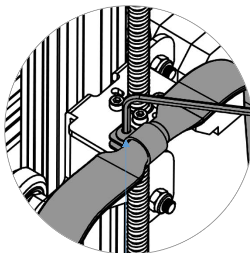
Винты M4 x 6
