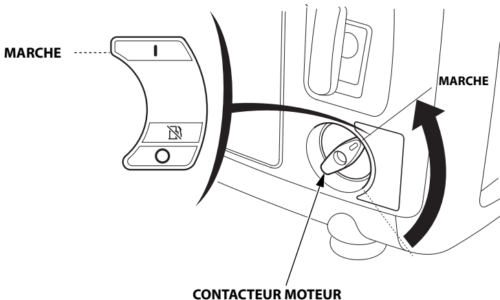
CONTACTEUR MOTEUR
