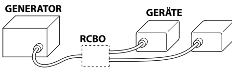
Anschluss an ein RCBO
