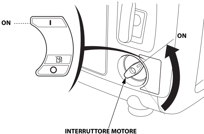
INTERRUTTORE MOTORE
