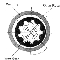
Gerotor
