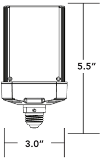
30W Model - E26
