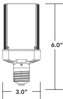
30W Model - E39
