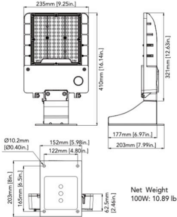
100W (Wall Mount)
