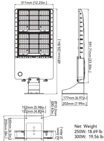
250W/300W (Wall Mount)
