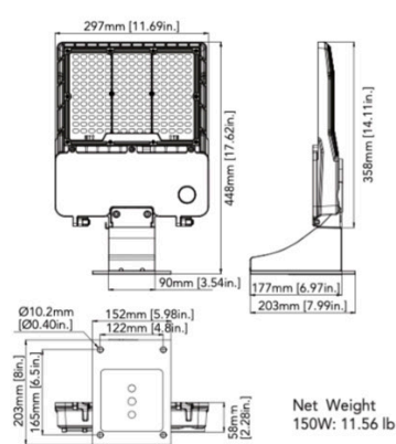
150W (Wall Mount)
