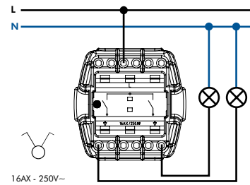
COMUTADOR DE ESCADA LUMINOSO
