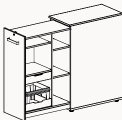
Höhe 1148 (3 OH), Breite 430, Tiefe 800/900/1000 mm
