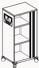
Höhe 1148 (3 OH), Breite 550, Tiefe 436 mm
