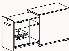
Höhe 740, Breite 430, Tiefe 800/900/1000 mm
