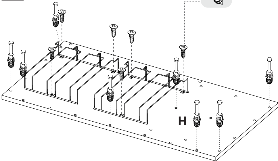
Tornillo lámina 6 X 9/16" Sheet Metal Screw
