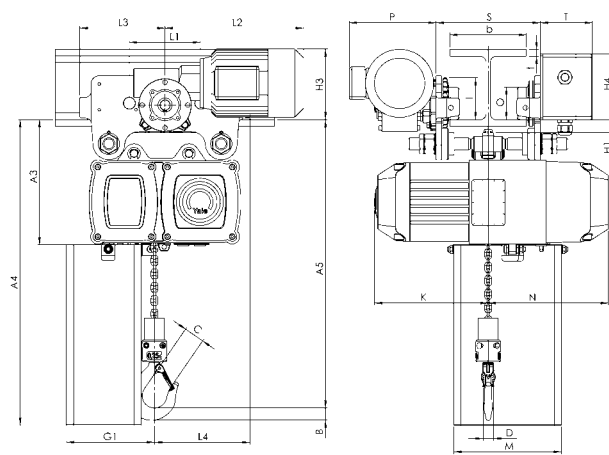
CPV/CPVF Festverbindung mit Elektrofahwerk
