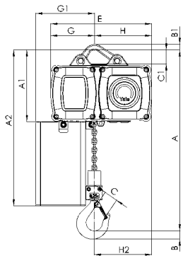
CPV/CPVF mit Aufhängebügel, 250 - 2.500 kg, einsträngig
