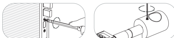
1. Retirez les vis de fixation et le cylindre d'origine
