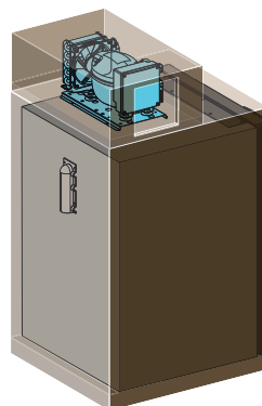
TOP
