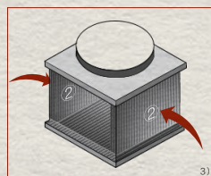
把两张②号碳布分别平放在内循环滤筒对称的两个侧面 注意：a边贴于①号碳布
