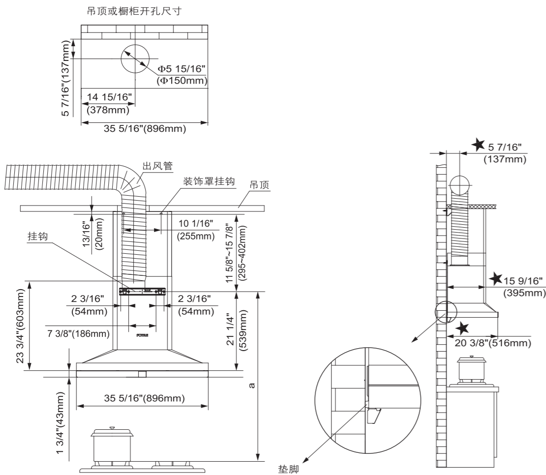
安装示意图 (★表示到墙的距离)
