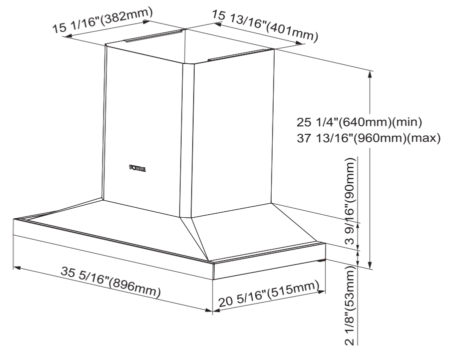
产品基本尺寸
