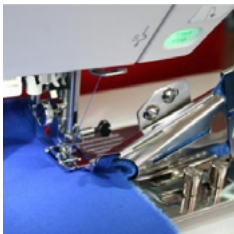
202-245-001 Dispositif pour pose de biais
