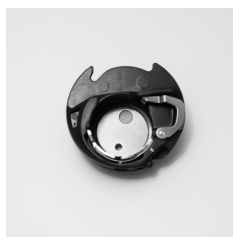
Capsule spéciale pour quilting mains-libres 200-445-029
