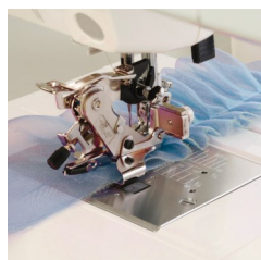
Appareil à plisser 846-415-031
