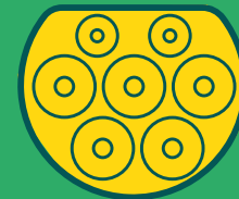
Type 2 Mennekes
