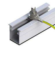
Befestigung des Erdungsdrahts mittels Hammerkopfschraube
