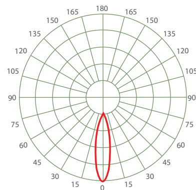
Curva fotométrica
