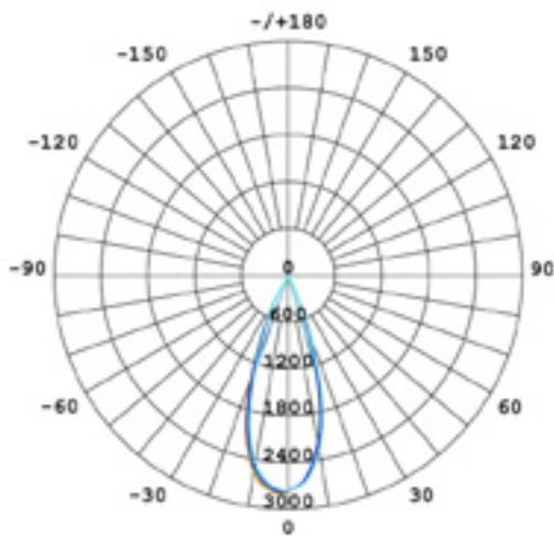
Curva fotométrica
