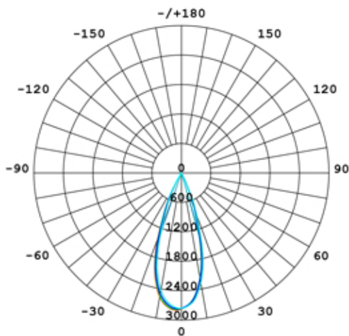
Curva fotométrica
