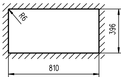
Ausschnitt Unterbau 1:20
