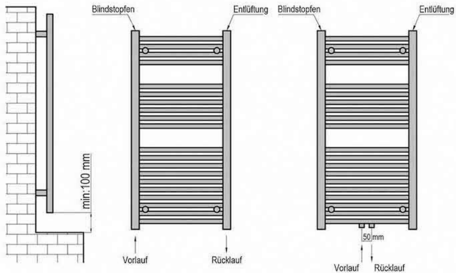
Seitenanschluss
