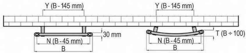
Seitenanschluss
