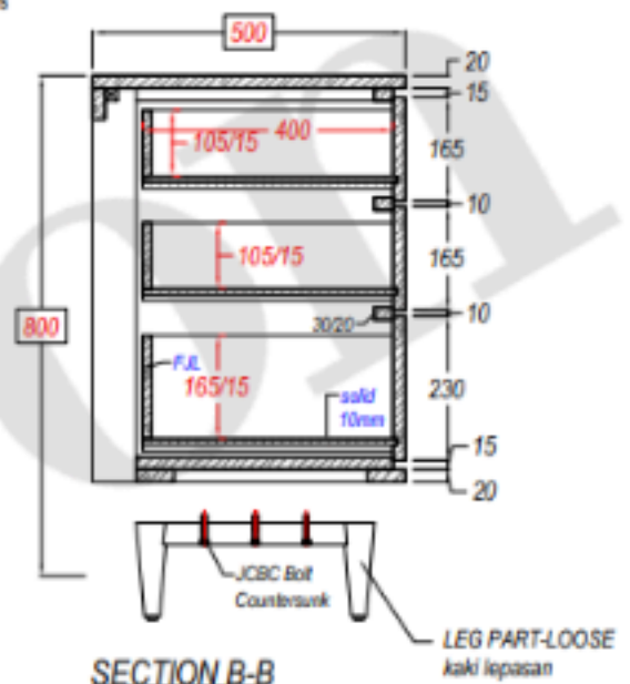
SECTION B-B Potongan B-B
