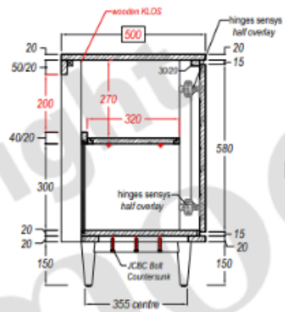
SECTION A-A Potongan A-A
