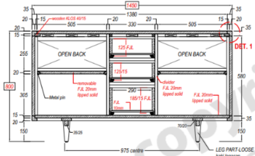
SECTION C-C Potongan C-C
