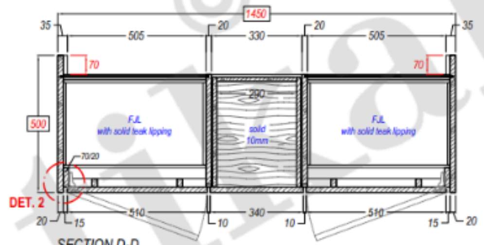
SECTION D-D Potongan D-D
