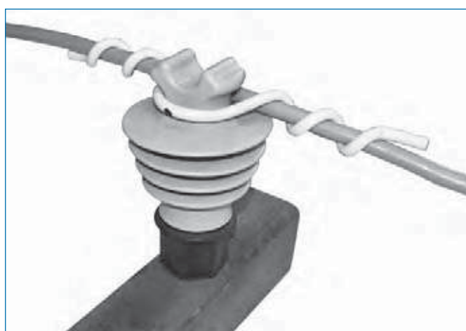
Aislador de Perno Fijo Ø Cuello = 57 mm
