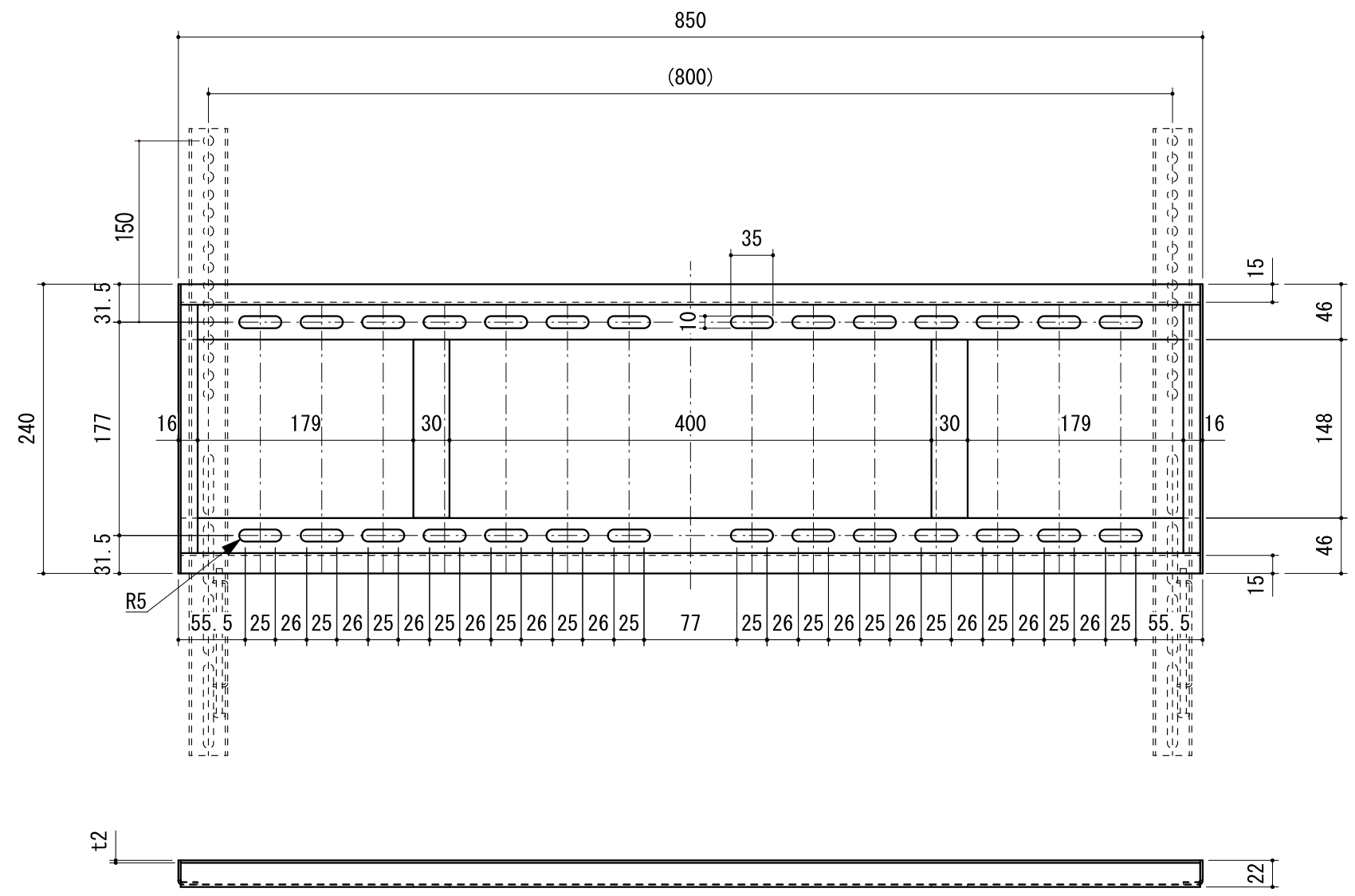
受け金具 奥行寸法
