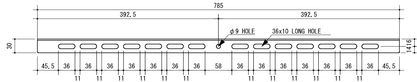
【平面図】
