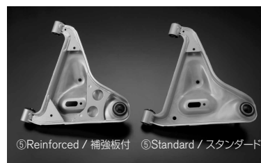
⑤ Reinforced / 補強板付 ⑥ Standard / スタンダード ⑤Rear A Arm / リヤAアーム
