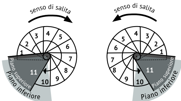
11 GRADINI pianerottolo incluso (11 ALZATE) Altezza tra i piani: Min. 231 cm - Max. 255 cm
