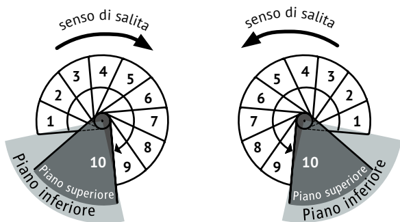
10 GRADINI pianerottolo incluso (10 ALZATE) Altezza tra i piani: Min. 210 cm - Max. 230 cm
