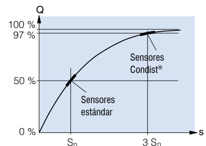
Fig. 3: Los sensores de la familia Extra Distance tienen una mayor distancia de detección, debido a la tecnología de oscilador Condist®
