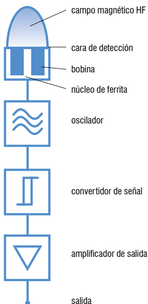
Fig. 1: Tecnología convencional de sensores inductivos, como la usada en la familia Classics
