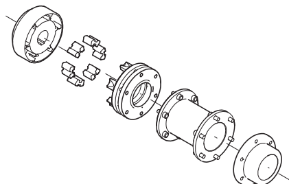
Fig. 24 Spacer coupling
