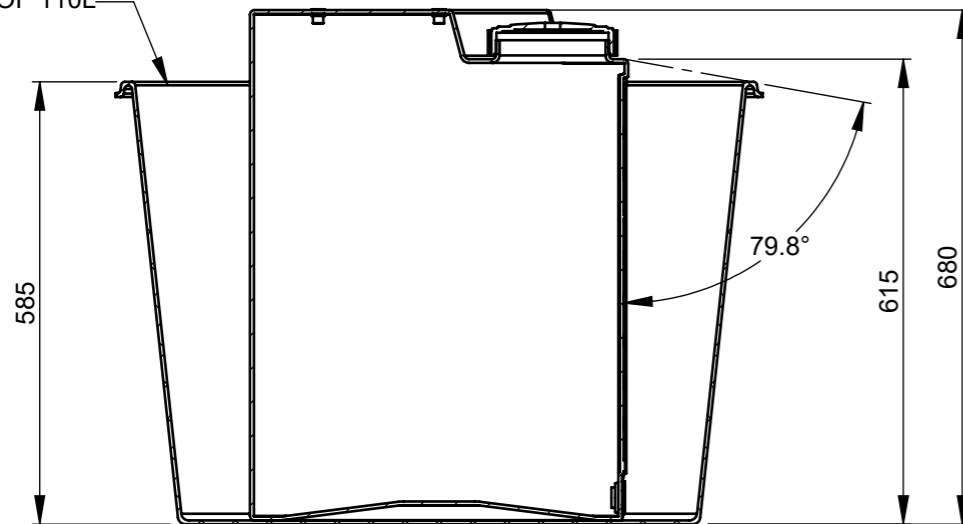
SECTION A-A
