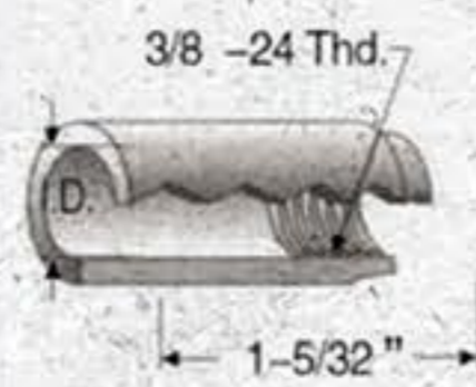
Alumina 1-5/32"
