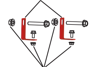
REMOVE THESE NUTS & BOLTS AS INDICATED. RETIRE LAS TUERCAS Y TORNILLOS COMO SE INDICA ENLEVEZ CES BOULONS ET ECROUS COMME INDIQUE
