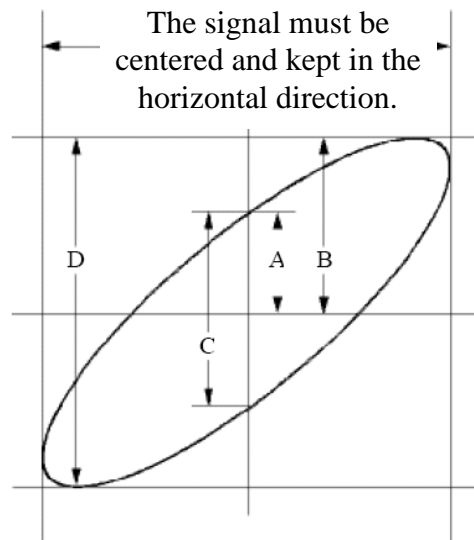
Fig.6-6 Lissajous Graph
