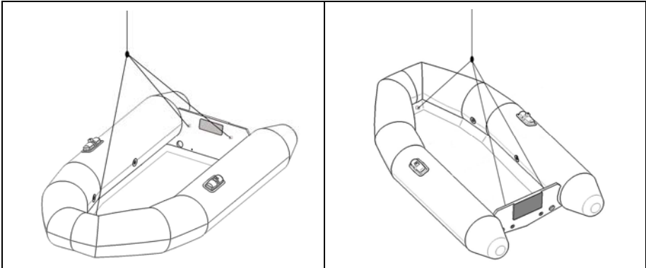
Punti di attacco per battelli con chiglia rigida
