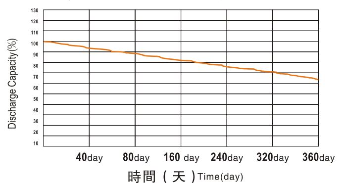
在常溫下LYP類電池的存儲特性曲線
