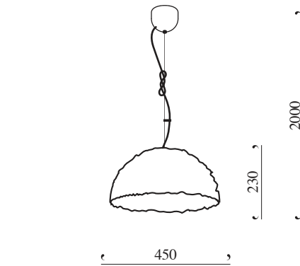
Pendant lamp / medium
