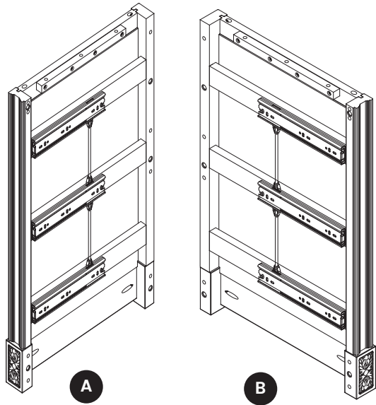
A Left Side x1 Lado izquierdo #43686
