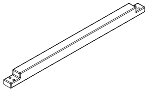
G Right Base Rail x 2 Barra base derecha x 2 42757
