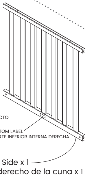
H Left Crib Side x 1 Costado izquierdo de la cuna x 1 42470
