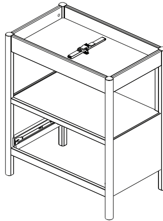
From Section 1: Step 3 Desde el Sección 1: paso 3
