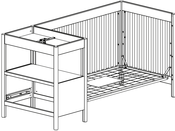
From Section 2: Step 5 Desde el Sección 2: paso 5
