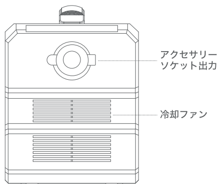
【本体背面】
